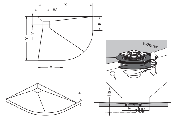
Rysunek przedstawia lewy wariant płyty
